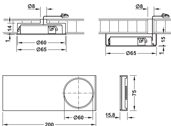
Díl pro montáž na strop
