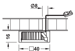
Montáž na strop, hranatý
