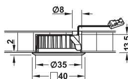
Zápusťná montáž, hranatý
