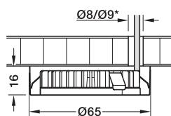
Montáž na strop, kulatý
