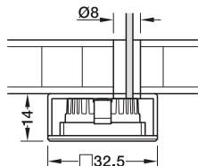
Montáž na strop, hranatý
