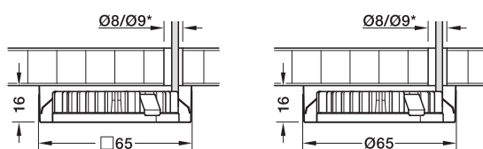
Montáž na strop, hranatý
