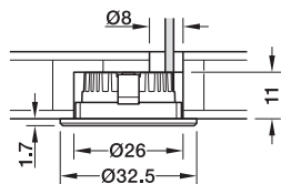
Zápusťná montáž, kulatý
