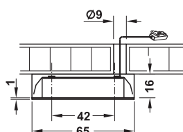
Montáž na strop
