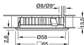
Zápusťná montáž, hranatý
