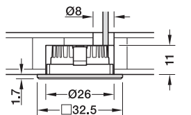
Zápusťná montáž, hranatý
