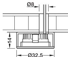
Montáž na strop, kulatý
