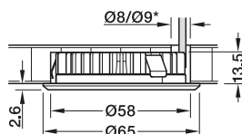
Zápusťná montáž, kulatý
