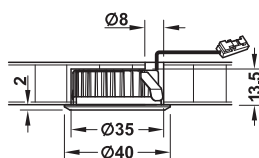
Zápusťná montáž, kulatý
