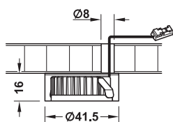
Montáž na strop, kulatý
